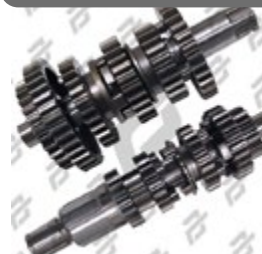
CAJA DE VELOCIDADES ENGRANE PRIMARIO Y SECUNDARIO
